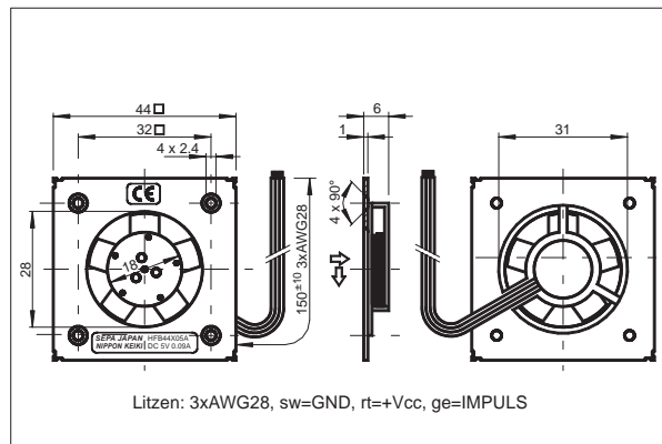
ABMESSUNGEN
