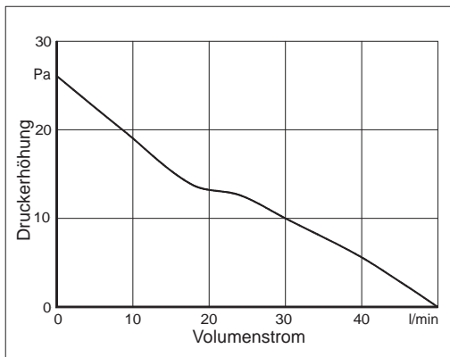
LÜFTERKENNLINIE
